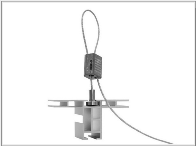
Stahlseilabhängiger für Profil mit Nut Länge 4 m bis 50 kg Traglast
